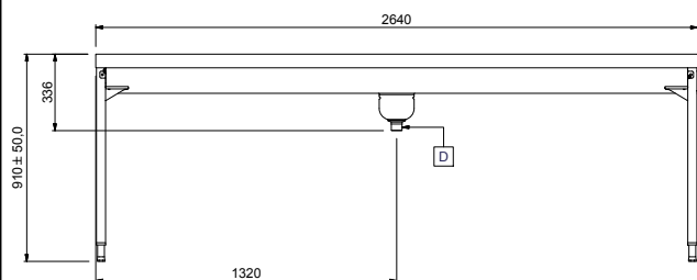
Boční
